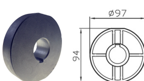
Polea 100 redonda | 61.005.022
